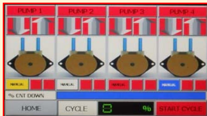
Visualizzazione funzionamento pompe
